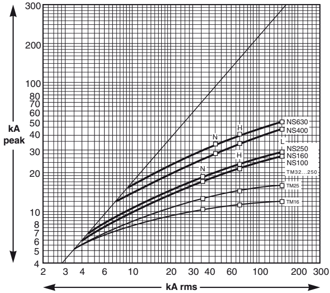
Compact NS100 - 630
